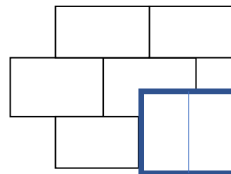
Posa corretta dei pannelli in prossimità di finestre o porte
